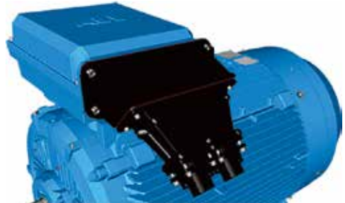
图4. 机座号315LKC, 355和400的接线盒，配备适配器和电缆密封端元件
