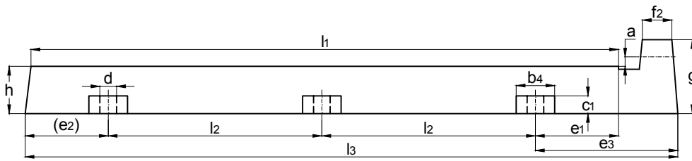
355-400 导轨
