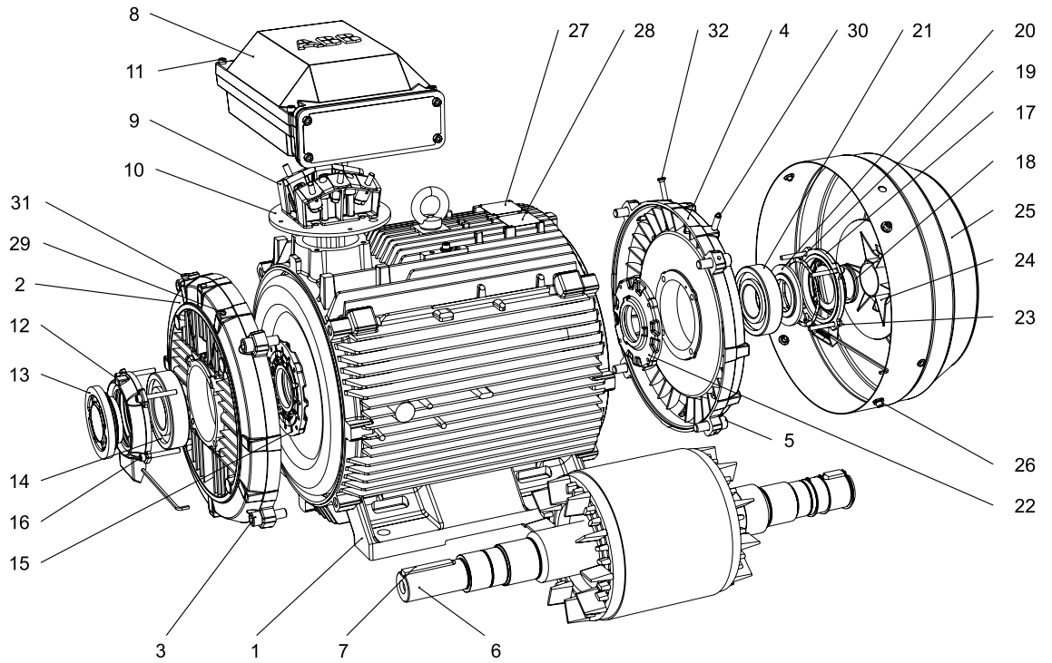
铸铁电机典型分解图，机座号315
