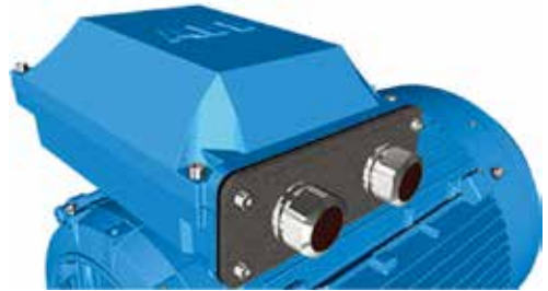
图3. 机座号280-315的接线盒(除LKC)，配备带螺纹孔的出线法兰
