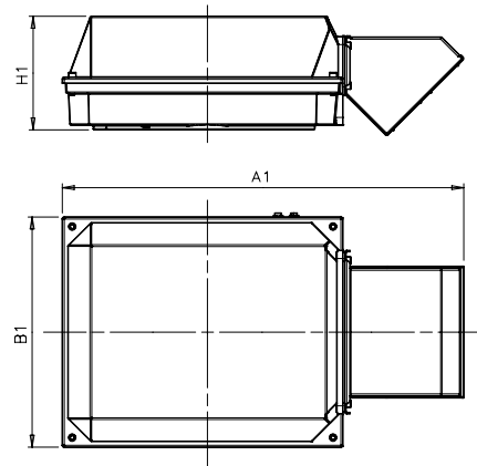
接线盒型号1200 + 适配器
